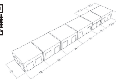
Dimensioni masselli
