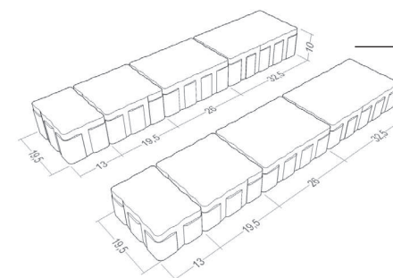
Dimensioni masselli
